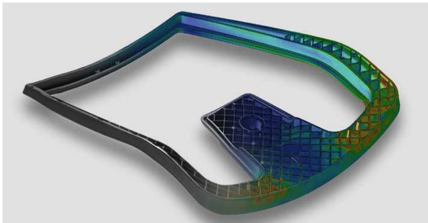
Simulazione di carico dello schienale in polipropilene (calcolo effettuato in base al metodo degli elementi finiti) Simulación de carga del respaldo de poliamida (Cálculo según el método de los elementos finitos)
